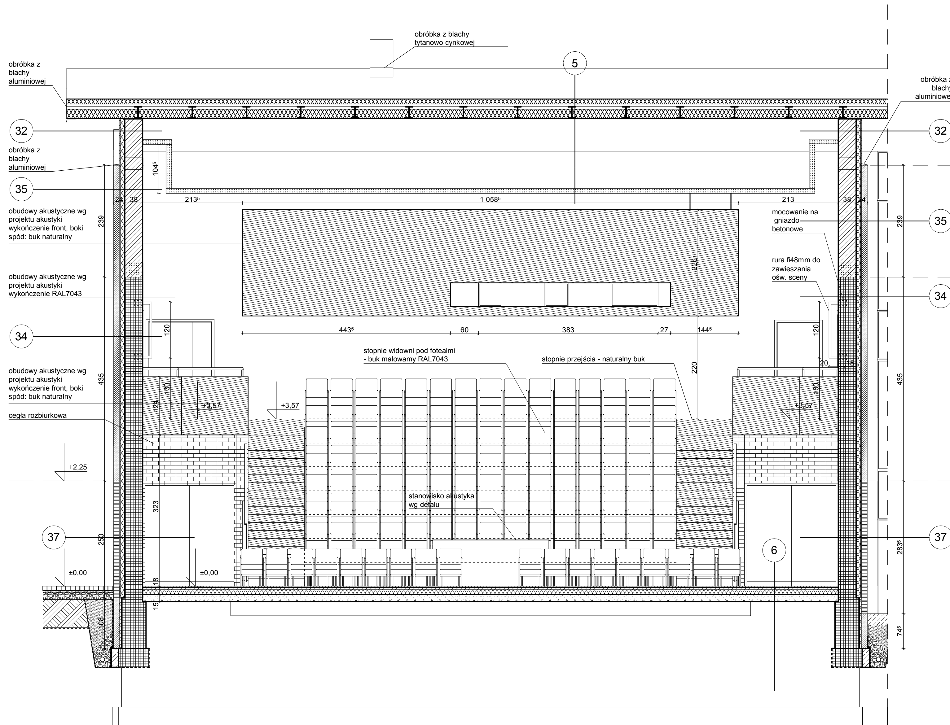
PRZEKROJ E-E
