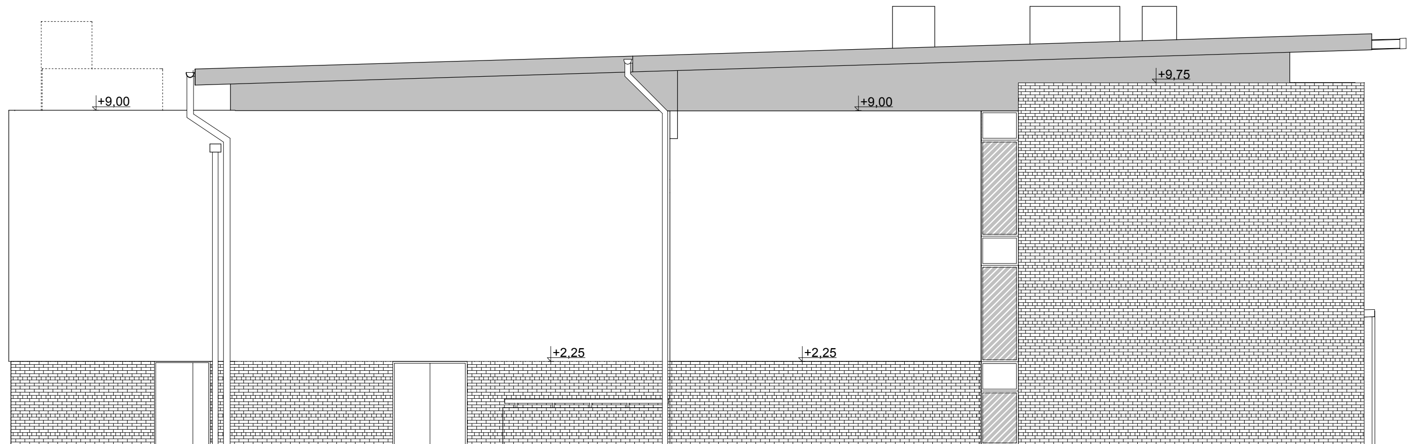
Elewacja północno-zachodnia
