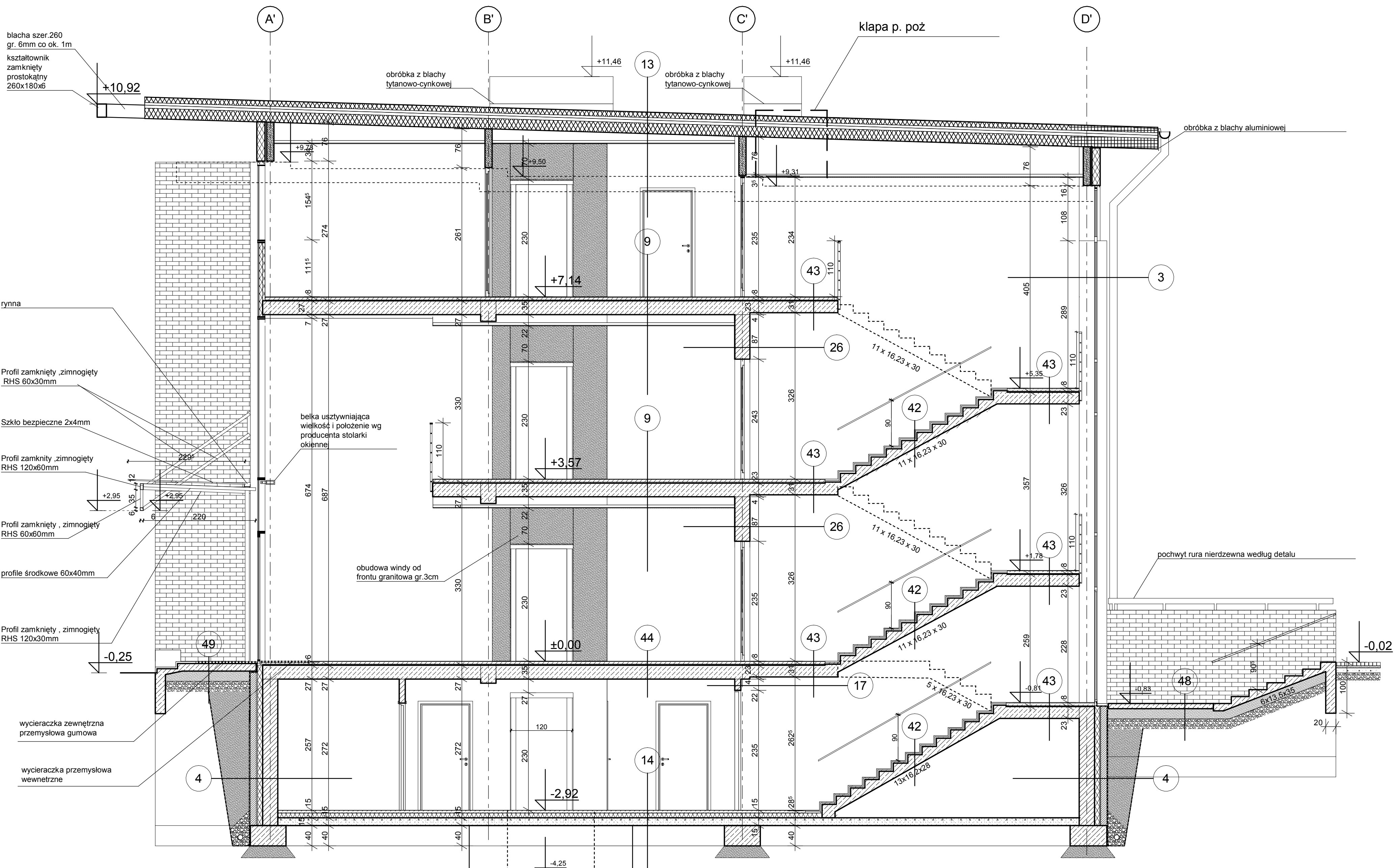
PRZEKROJ B-B
