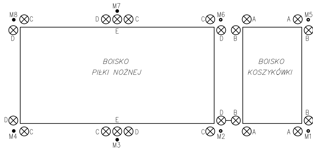
ROZMIESZCZENIE MASZTÓW I PROJEKTORÓW
