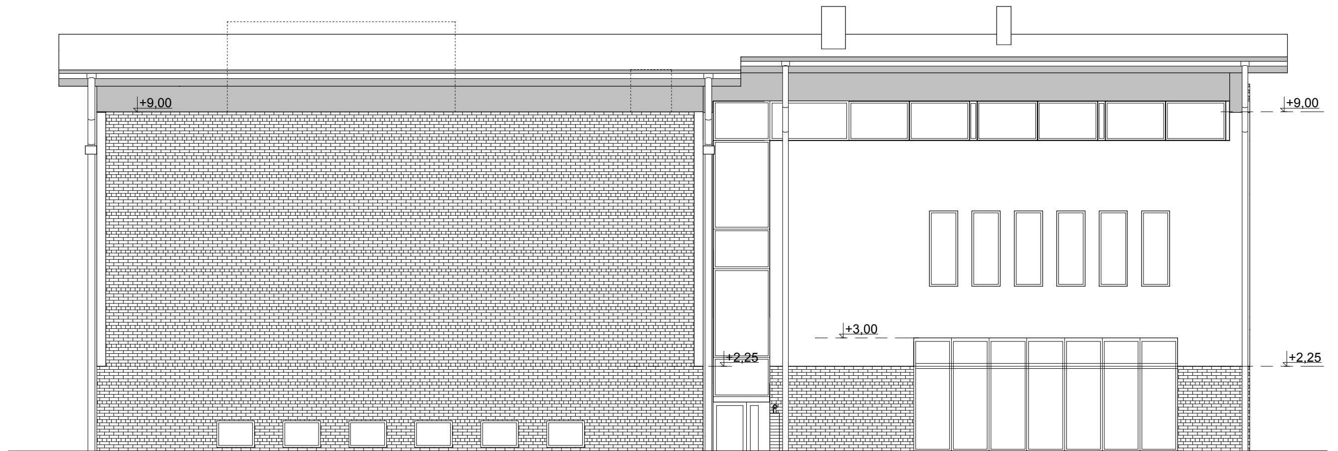
Elewacja północno-wschodnia
