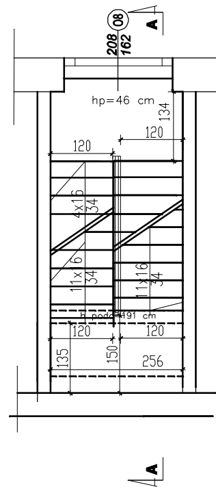
PRZEKRÓJ II-II
