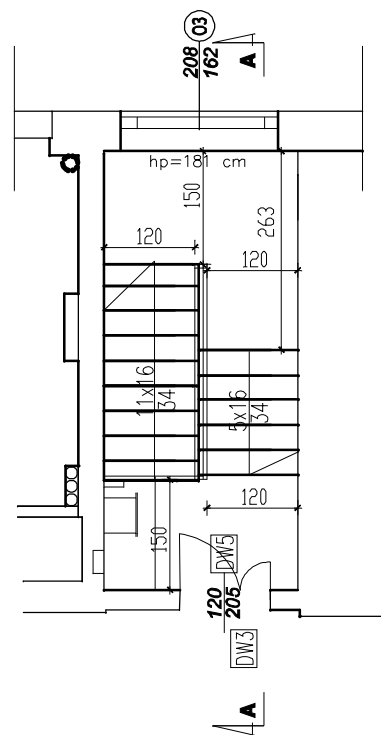
PRZEKRÓJ III-III
